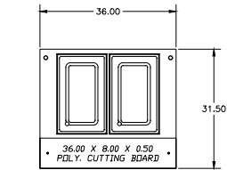
Plan View EHEI36C, EHEI36C-208
