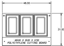
Plan View EHEI48C
