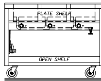
Elevation View EHEI48C
