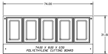
Plan View EHEI74C
