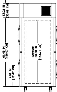
TYP. LEFT END VIEW
