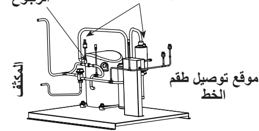
توصيل طقم عداد متشعب أو خرطوم مزود بضاغطات لقلب الصمام عند طرفيه
