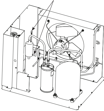
التوصيلات البديلة لصمامات شريدنر بوحدة التكتيف
