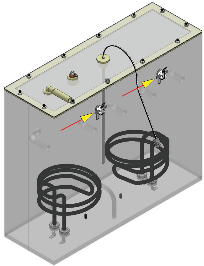
FIG. 18-2 LIMIT THERMOSTATS
